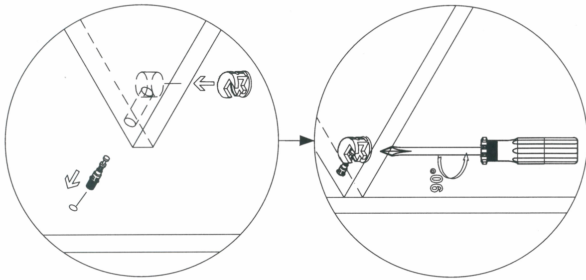
Rys. 1 Schemat złącza mimośrodowego
