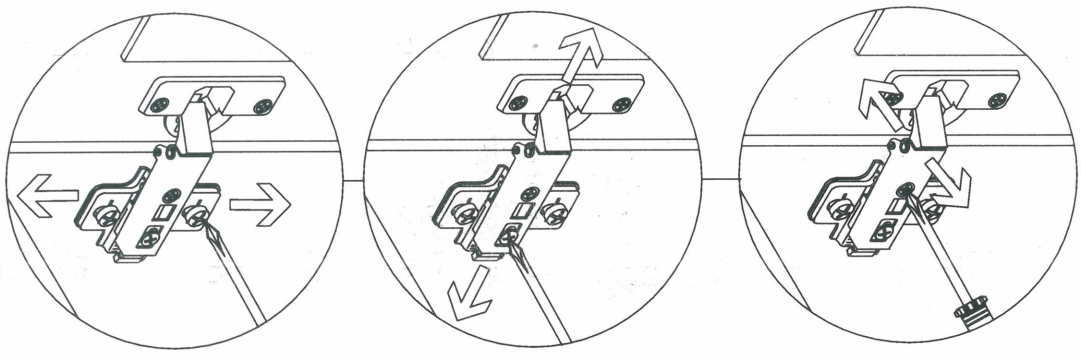
Regulacja ustawień drzwiczek.
